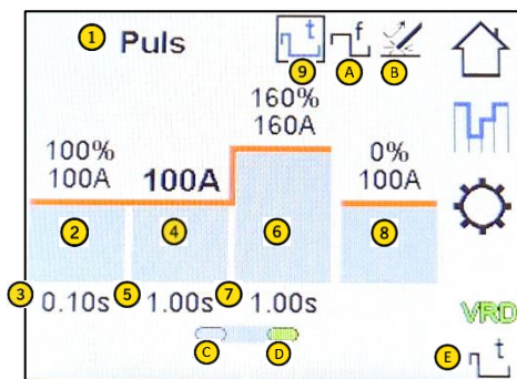
Fig. 3: Curva di corrente
